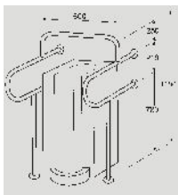
▲ A61-620 不銹鋼小便斗扶手 W698xH1196mm
